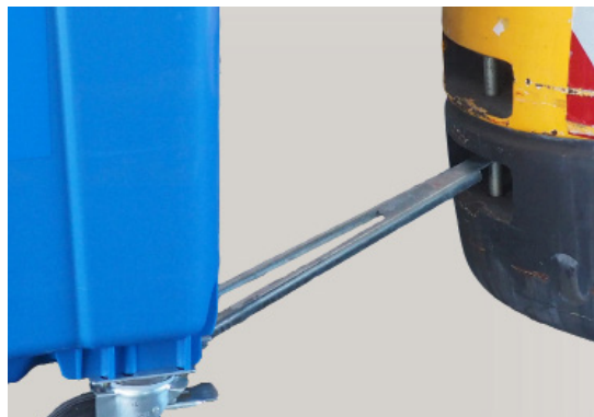
Deichsel des Müllbehälters an der Dornkupplung der Zugmaschine
